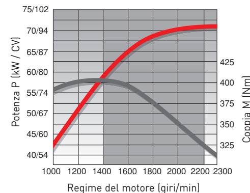
CURVA DI POTENZA DEL QUANTUM C
